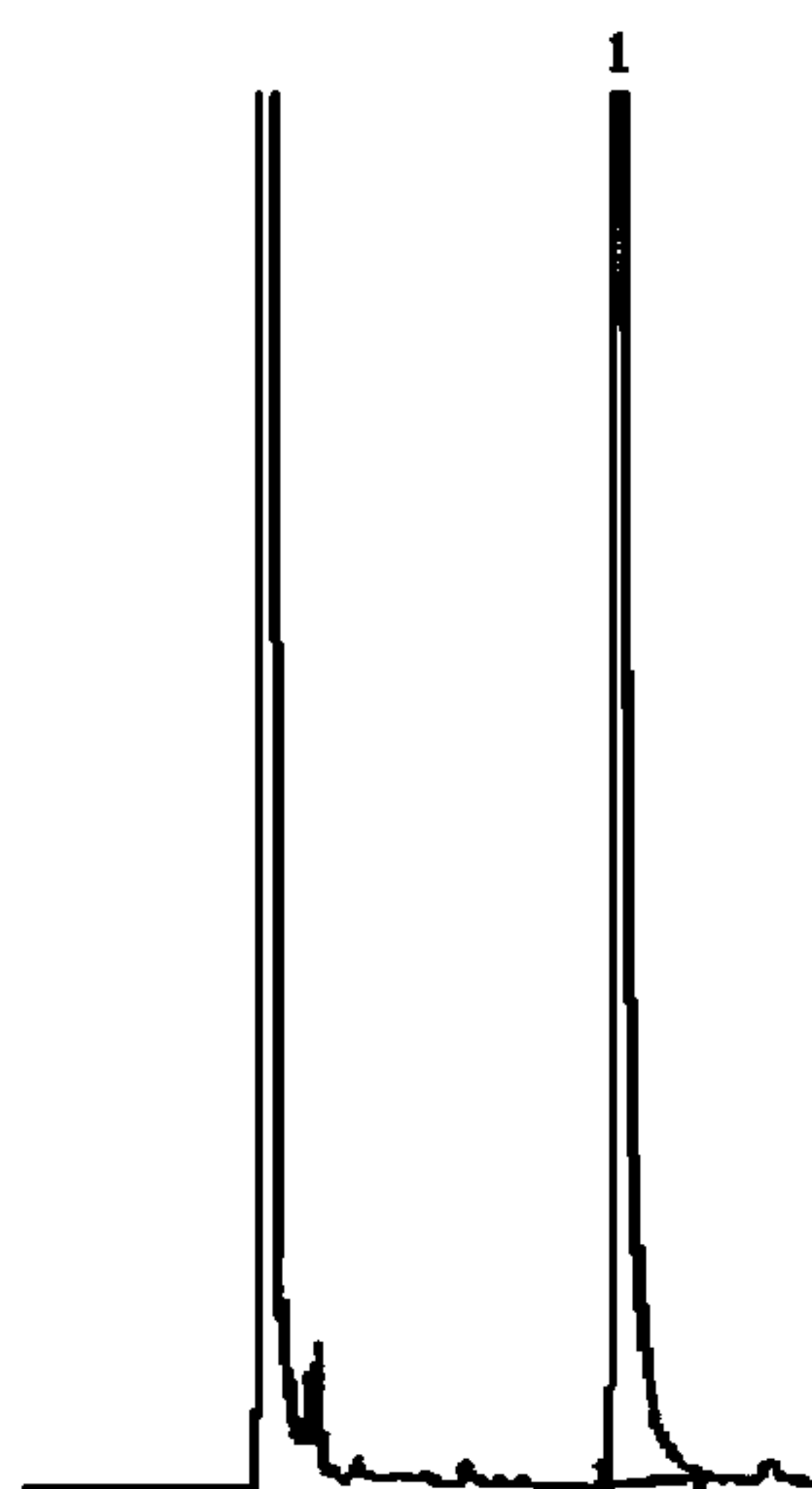
图 A.1 40%乙烯利水剂甲酯化产物的气相色谱图
