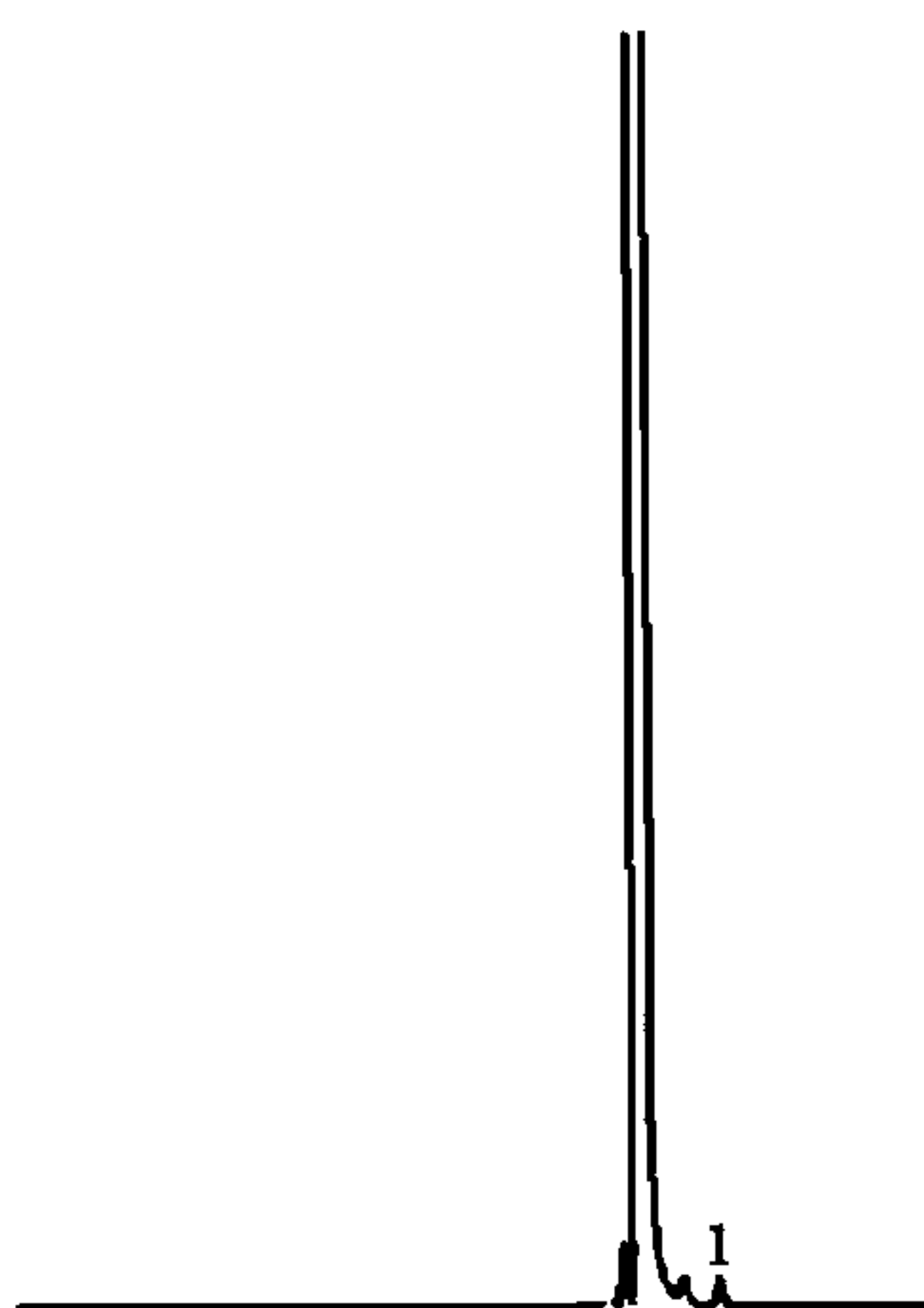
图 1 40%乙烯利水剂中 1,2-二氯乙烷测定的气相色谱图
